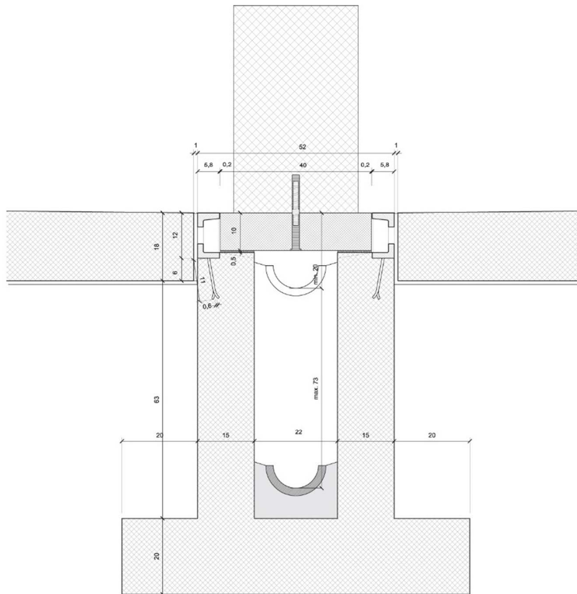
COUPE SUR CANIVEAU ET BORNE 1:5
